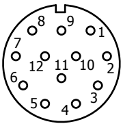
Stekeraanzicht (buitenaanzicht)
