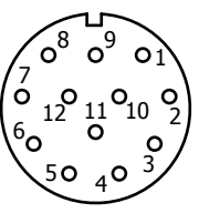
Stekeraanzicht (buitenaanzicht)
