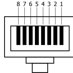
RJ45
