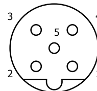
KBL031-xxx 5P M12 Female B-Gecodeerd
