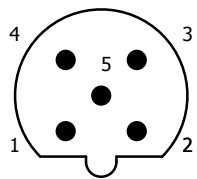
KBL032-xxx 5P M12 male/female B-Gecodeerd
