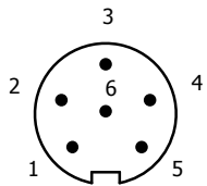
Stekeraanzicht (buitenaanzicht)
